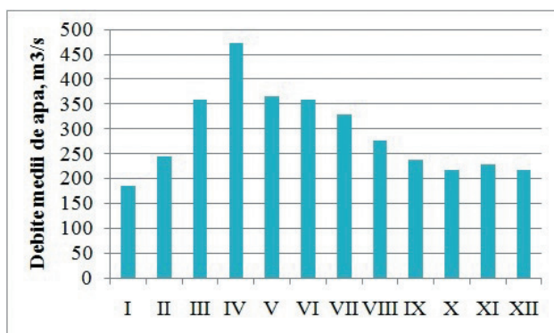
Figura 1.20 Debitul mediu lunar al fluviului Nistru, p. Dubăsari
