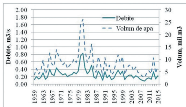
Figura 1.23 Debitele medii anuale și volumele scurgerii râului Cogîlnic, p. Hîncești
