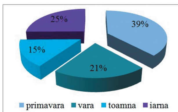
Figura 1.25 Repartiția scurgerii de apă pe anotimpuri, râul Cogîlnic, p. Hîncești
