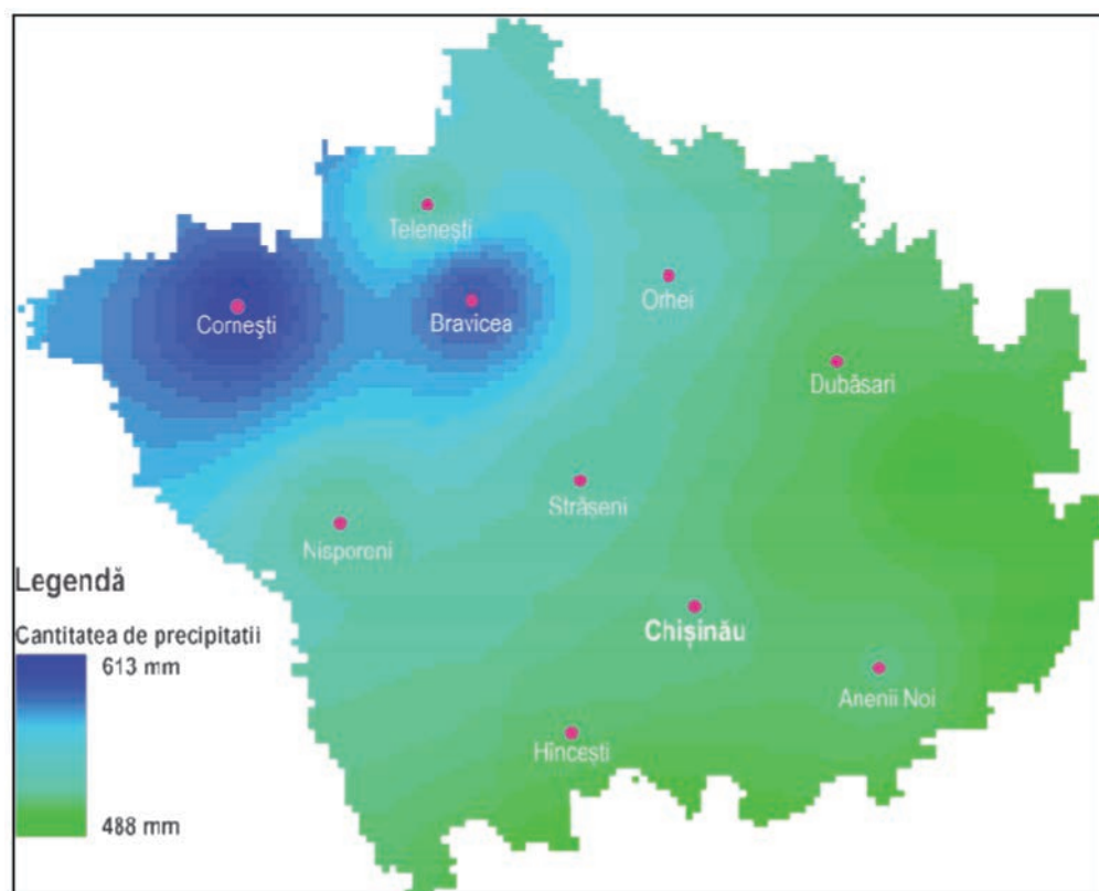
Fig. 1.14 Repartiția cantității medii anuale de precipitații pe teritoriul RD Centru (în perioada 1981-2017)
