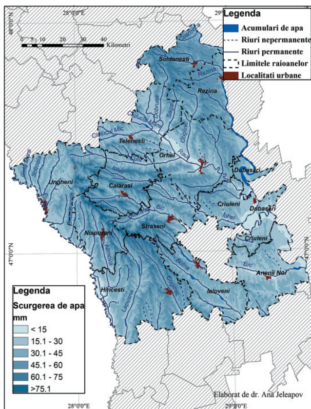
Fig. 1.28 Scurgerea de apă în RD Centru [59]
