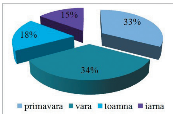
Figura 1.19 Repartiția scurgerii de apă pe anotimpuri, râul Prut, postul Ungheni
