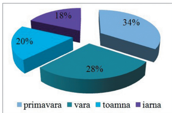
Figura 1.18 Repartiția scurgerii de apă pe anotimpuri, fluviul Nistru, postul Dubăsari
