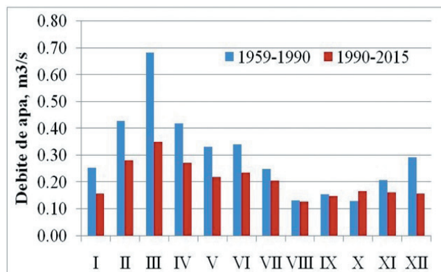
Figura 1.27 Debitele medii lunare ale râului Cogîlnic p. Hîncești (calculat în baza datelor SHS)
