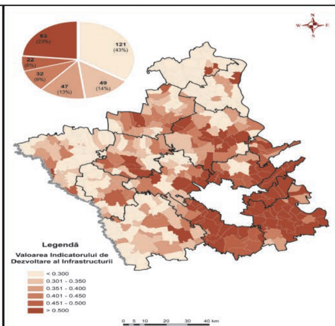
Fig. 3.19 Indicele agregat al componentei infrastructură
