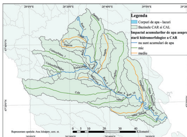
Fig. 4.19 Impactul acumulărilor de apă asupra stării hidromorfologice a CAR
