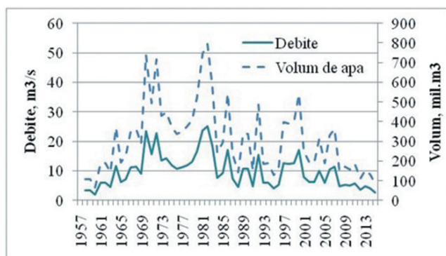
Figura 1.22 Debitele medii anuale și volumele scurgerii râului Răut, p. Jeloboc
