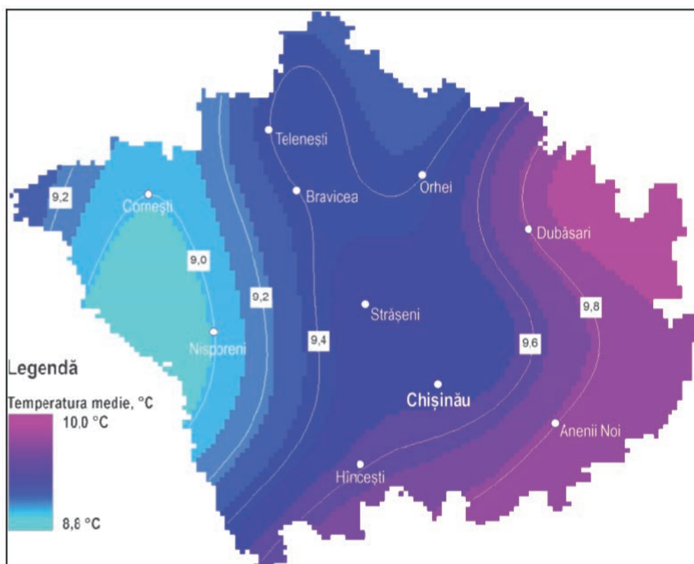
Fig. 1.13 Repartiția temperaturii medii anuale a aerului pe teritoriul RD Centru (perioada anilor 1981-2017)
