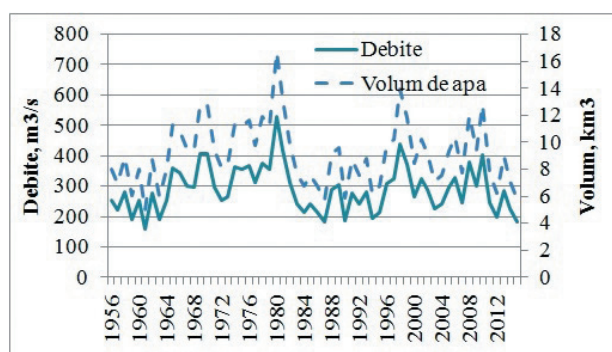
Figura 1.16 Debitelor medii anuale și volumele scurgerii de apă ale fluviului Nistru, postul Dubăsari (calculat în baza SHS)
